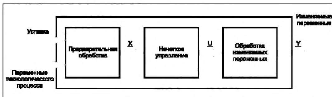
Рисунок А.13а — Основанный на нечетком управлении контроллер: базовая структура
